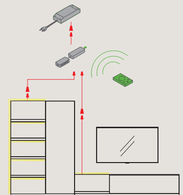
Ejemplo instalación controlador mando a distancia 1 canal [para encender al mismo tiempo 1 conjunto con luz].
