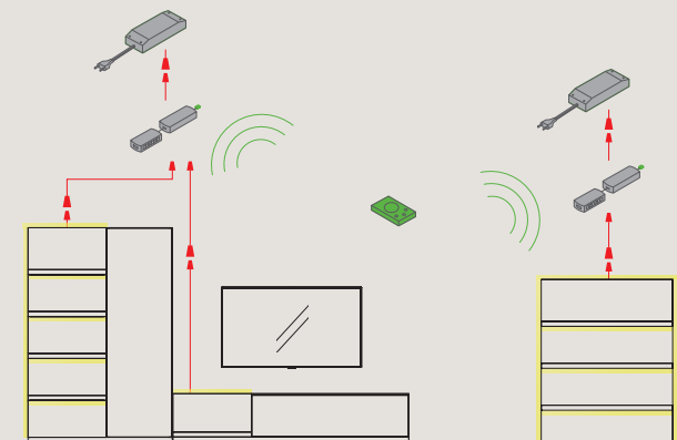
Ejemplo instalación controlador mando a distancia 4 canales [para encender individualmente hasta 4 conjuntos con luz].
