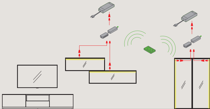
Ejemplo instalación controlador mando a distancia 4 canales (para encender individualmente hasta 4 conjuntos de módulos con luz).
