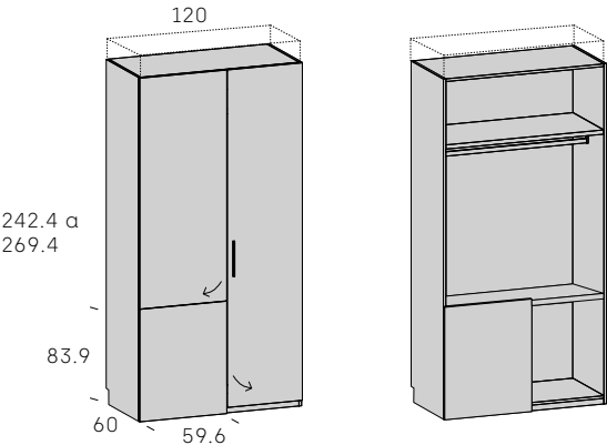
Armario con plafón inferior ciego IZQUIERDA
