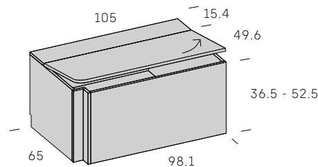
Arcón Complet rincón fondo 65 DERECHA
