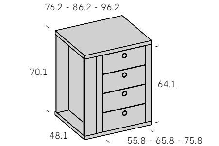
Cajonera interior 4 cajones para armario de puertas PLEGABLES
