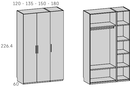
Armario 3 puertas DERECHA
