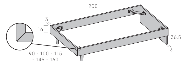
Aro Miter con patas de madera
