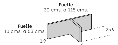
Soporte fuelle ancho y alto
