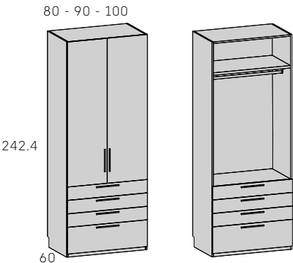
Armario 2 puertas + 3 cajones + 1 cajón doble
