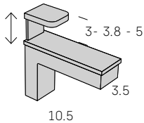
Soporte Quadra aluminio para estante pared
