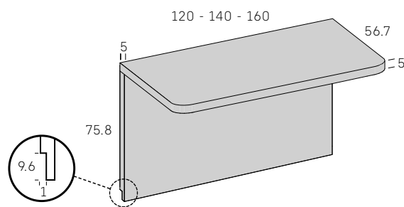
Escritorio Square cantos curvos
