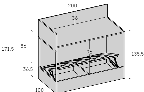
Litera Aken somier elevable IZQUIERDA
