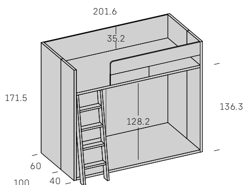
Litera Mixed tarima DERECHA con guardamiedos y escalera
