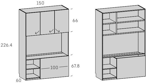
Armario altillo 3 puertas + hueco + arcón DERECHA
