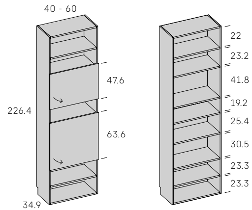
Librería Troya 2 puertas 47.6 + 63.6 cms. DERECHA
