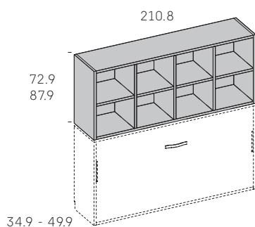
Estantería horizontal para abatible horizontal 1 cama s/ 135 - 150
