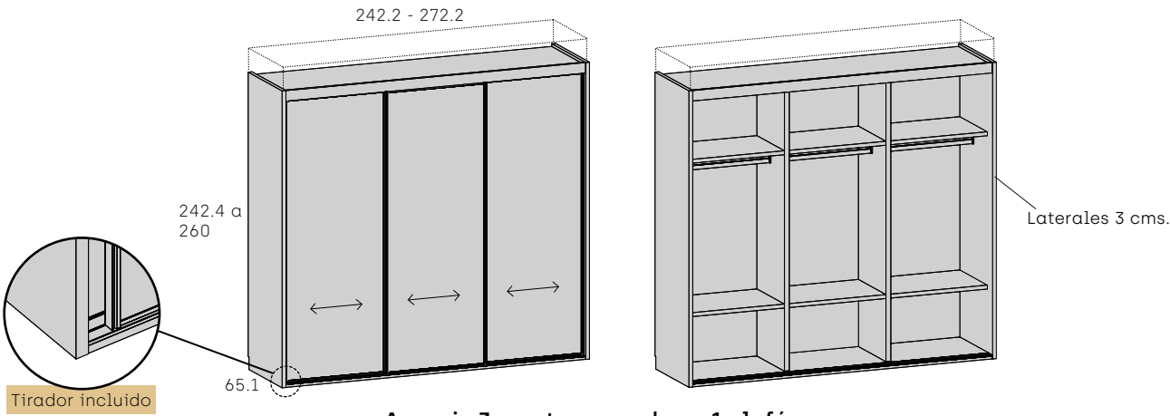
Armario 3 puertas correderas 1 plafón
