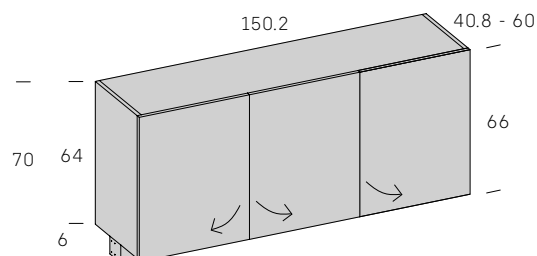
Altillo puente 3 puertas
