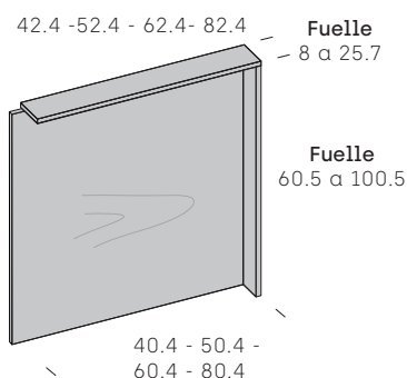
Ala cabezal XYZ DERECHA
