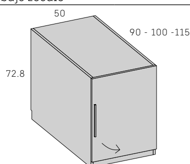
Arcón 1 puerta DERECHA
