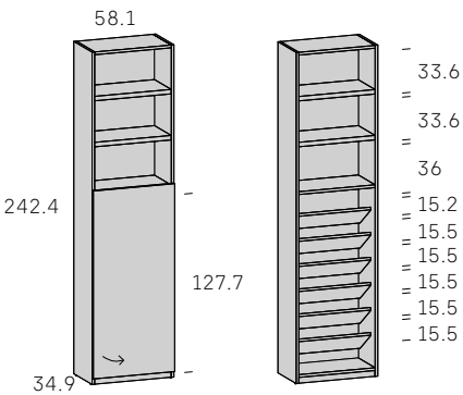
Armario terminal zapatero DERECHA
