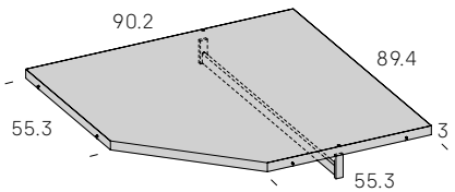
Estante interior con barra para armario rincón DERECHA
