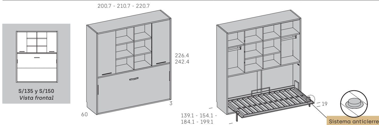
Abatible horizontal 1 cama + 2 puertas + estantería central
