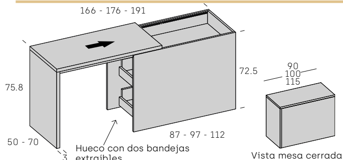
Arcón - Escritorio extraíble con cajones
