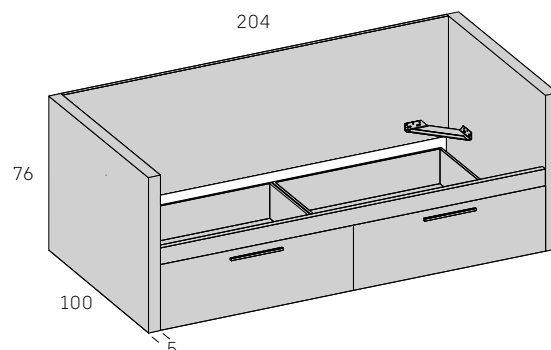
Nido alto Basic 2 cajones con ruedas. Laterales de 5 cms.
