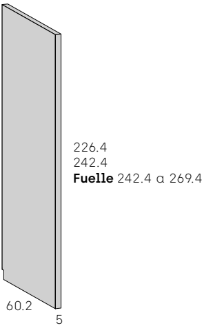
Sobrecostado armario 5 cms.
