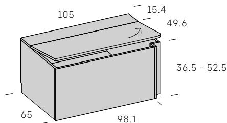
Arcón Complet rincón fondo 65 IZQUIERDA
