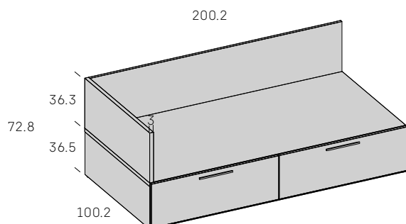
Nido It 2 cajones alto 36.5 cms. Cierre IZQUIERDA
