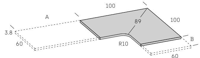
Sobre rincón de 60 cms. especial
