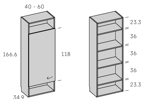
Librería Troya 1 puerta 118 cms. IZQUIERDA
