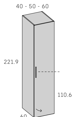
Armario Complet 1 puerta DERECHA 221.9
