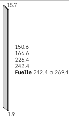
Montante Columna rincón curvo
