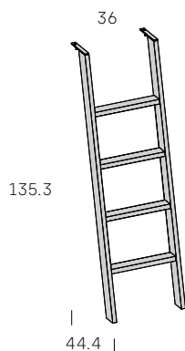
Escalera metal Block a suelo
