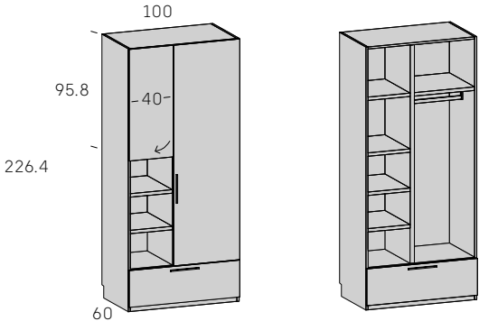
Armario asimétrico 1 puerta altillo IZQUIERDA + huecos + puerta DERECHA + 1 cajón doble
