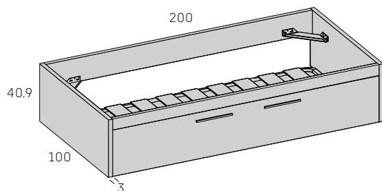
Nido Basic arrastre. Laterales de 3 cms.
