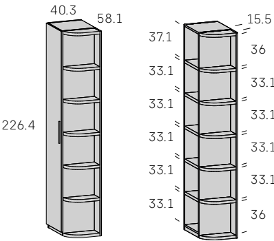
Armario terminal zapatero IZQUIERDA
