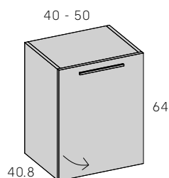
Módulo 1 puerta derecha
