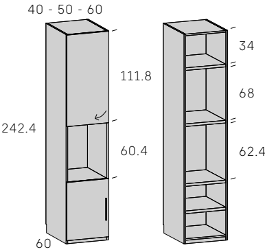
Armario 1 puerta IZQUIERDA + hueco + 1 puerta IZQUIERDA
