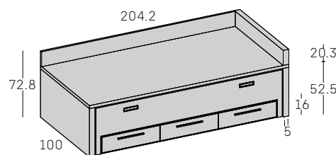
Compacto DUO 2 camas + 3 cajones. Cierre recto der. 5 cms. grueso
