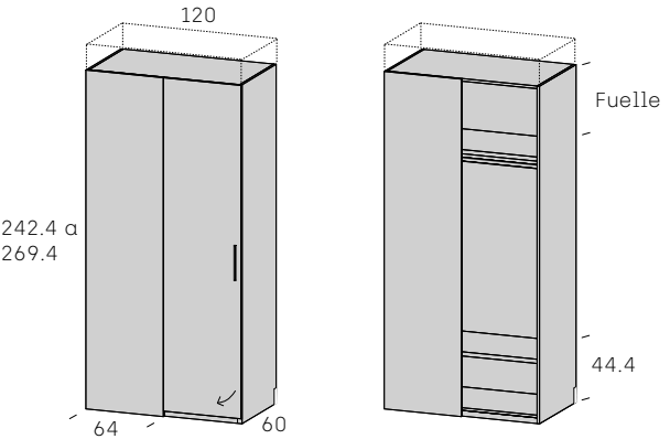
Armario ciego 1 puerta DERECHA
