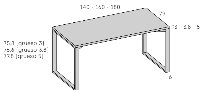
Mesa despacho patas Quadro
