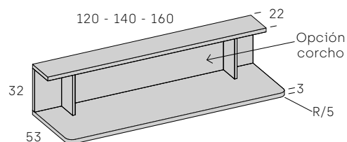
Escritorio Muse cantos curvos
