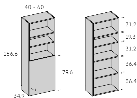
Librería Troya 1 puerta inferior 79.6 cms. DERECHA
