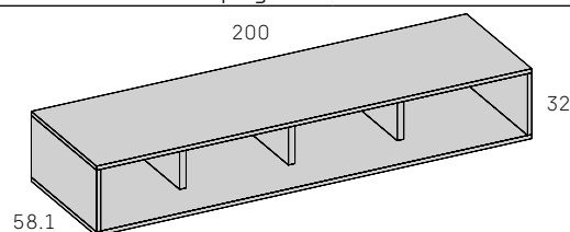
Cubo Complet con 3 partidores
