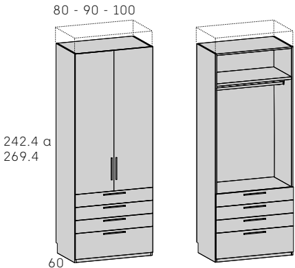
Armario 2 puertas + 3 cajones + 1 cajón doble
