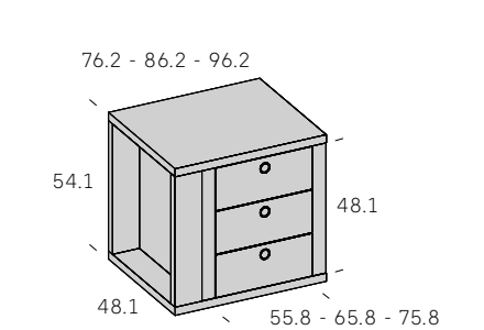
Cajonera interior 3 cajones para armario de puertas PLEGABLES
