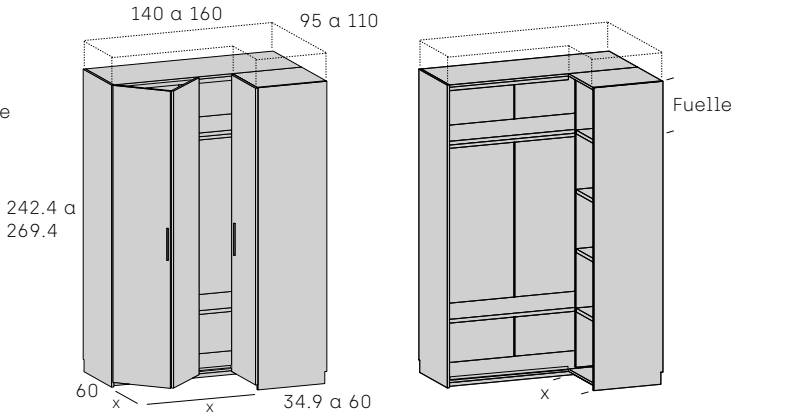
Armario p. plegables - batiente adaptable DERECHA especial
