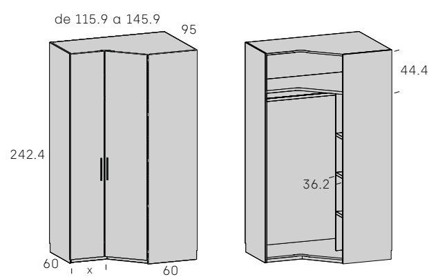
Armario recto - recto IZQUIERDA especial
