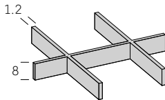
Organizador interior para cajoneras interiores
