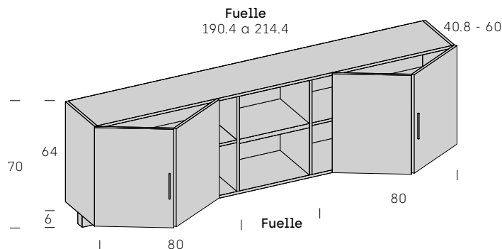
Altillo puente 4 puertas + hueco central Fuelle
