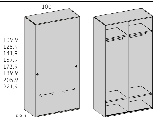
Armario Complet 2 puertas correderas ancho 100
