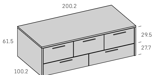
Compacto Praktic 2 cajones con guías + 3 cajones alto 29.5 cms.
