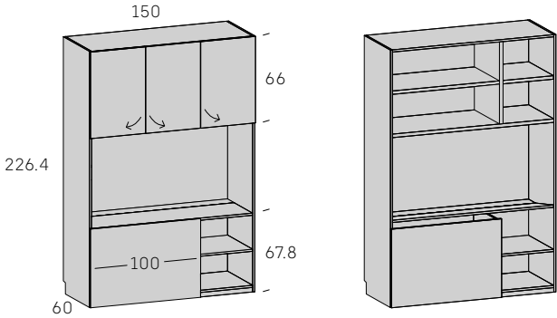
Armario altillo 3 puertas + hueco + arcón IZQUIERDA
