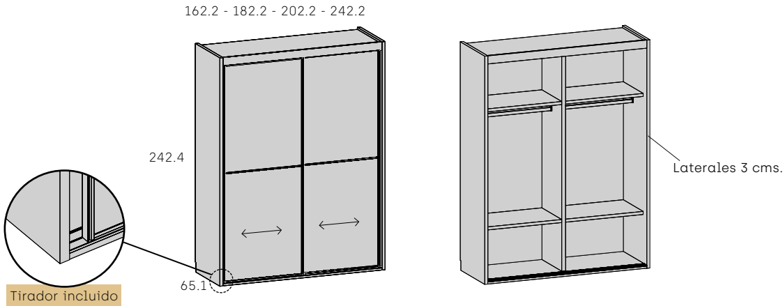
Armario 2 puertas correderas 2 plafones
