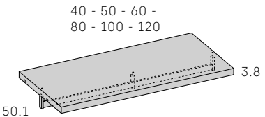
Estante interior con barra vestidores ADD
