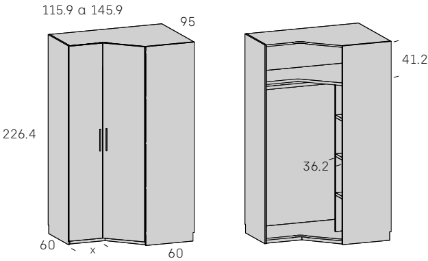
Armario recto - recto IZQUIERDA especial
