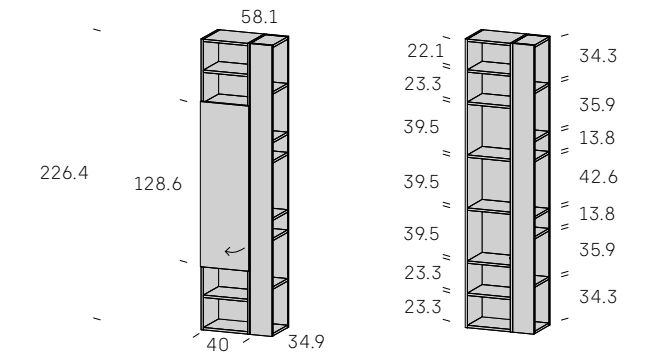
Terminal Troya armario IZQUIERDA
