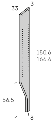
Montante Forma IZQUIERDO
