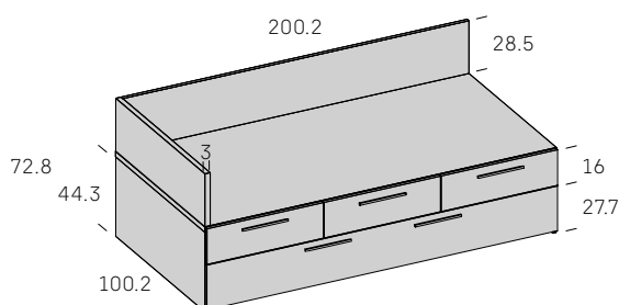
Compacto It 1 arrastre + 3 cajones alto 16 cms. Cierre izquierda
