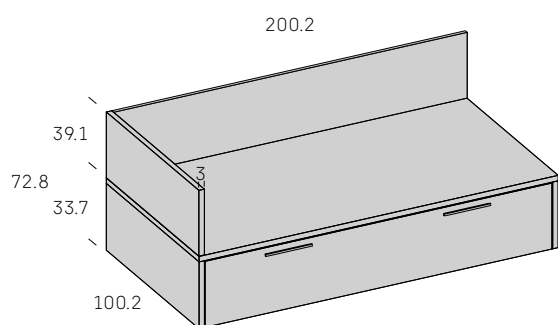
Nido Praktic arrastre alto 33.7 cms. Cierre izquierda
