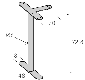
Soporte mesa pata Hype
