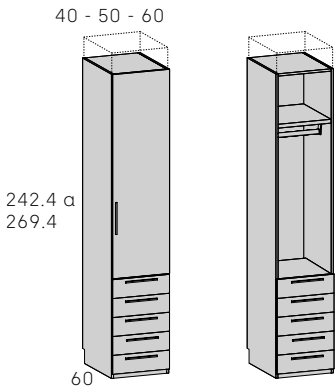
Armario 1 puerta DERECHA + 5 cajones
