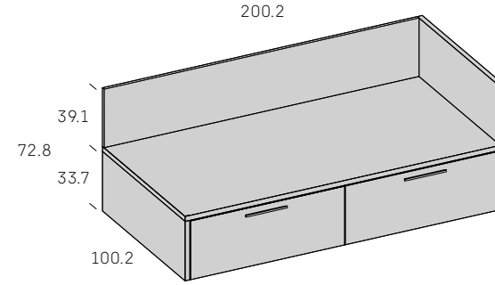
Nido Praktic 2 cajones alto 33.7 cms. Cierre DERECHA
