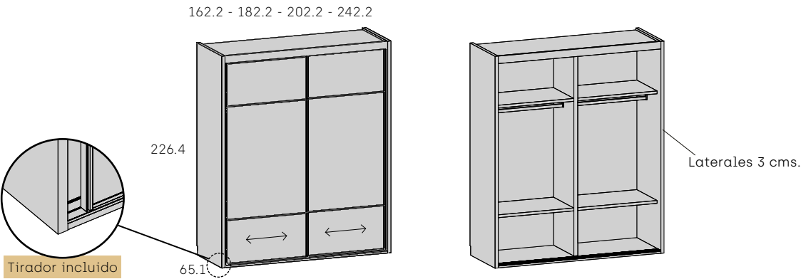
Armario 2 puertas correderas 3 plafones
