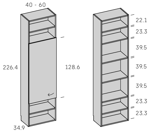
Librería Troya 1 puerta 128.6 cms. IZQUIERDA
