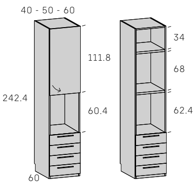
Armario 1 puerta DERECHA + hueco + 4 cajones
