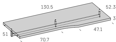
Estante interior con barra para armario recto - recto IZQUIERDA
