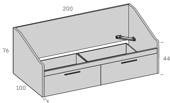
Nido Siena 2 cajones con ruedas. Laterales de 3 cms.
