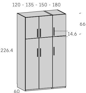
Armario 3 puertas + altillo 3 puertas DERECHA
