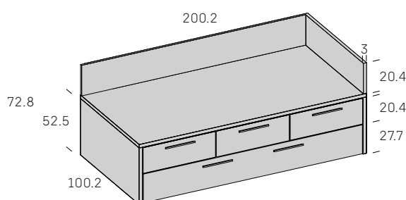
Compacto Praktic 1 arrastre + 3 cajones alto 20.4 cms. Cierre derecha
