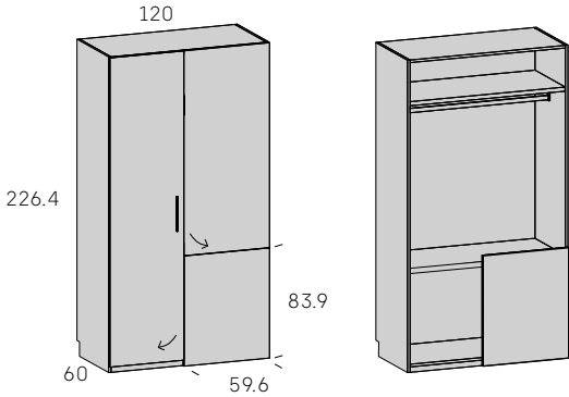
Armario con plafón inferior ciego DERECHA
