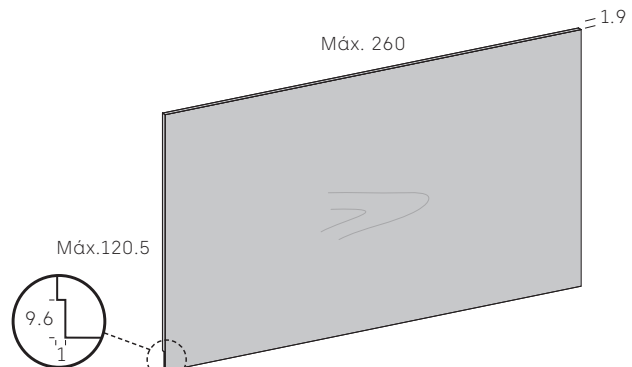
Panel recto especial grueso 1.9 cms. para zócalo
