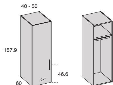
Armario Complet 1 puerta IZQUIERDA 157.9
