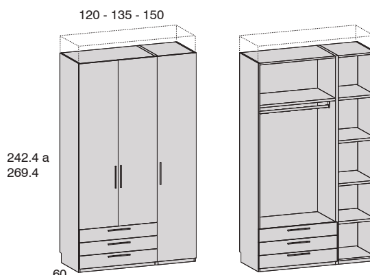
Armario 3 puertas DERECHA + 3 cajones
