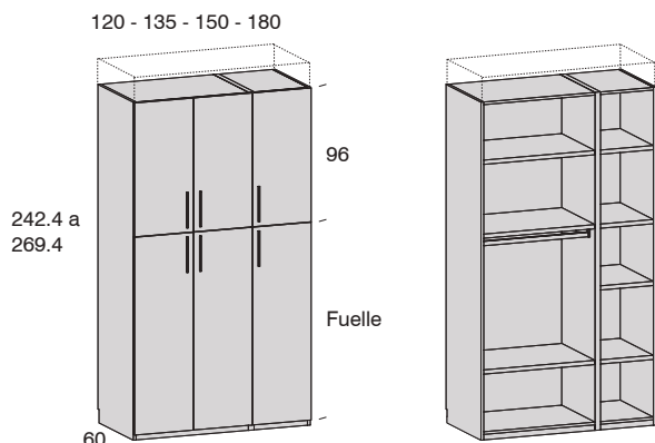
Armario 3 puertas + altillo 3 puertas DERECHA
