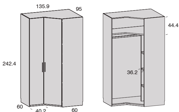
Armario recto - recto IZQUIERDA
