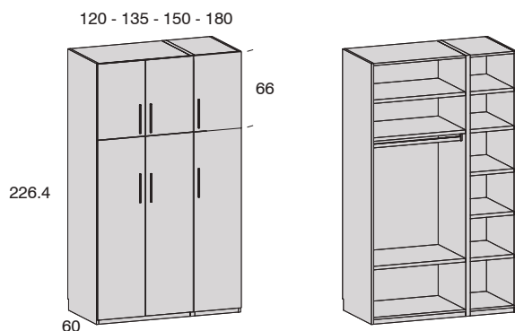
Armario 3 puertas + altillo 3 puertas DERECHA
