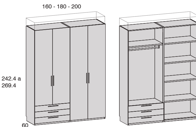
Armario 4 puertas DERECHA + 3 cajones
