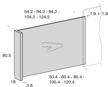
Ala Bodja IZQUIERDA
