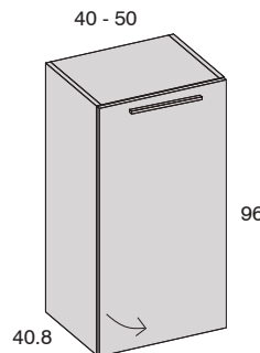
Módulo 1 puerta DERECHA
