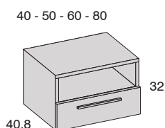
Mesita 1 cajón + hueco
