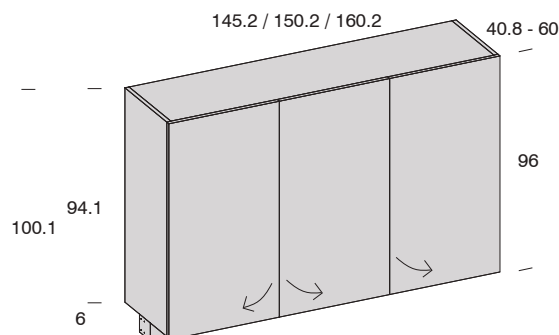
Altijo puente 3 puertas batientes
