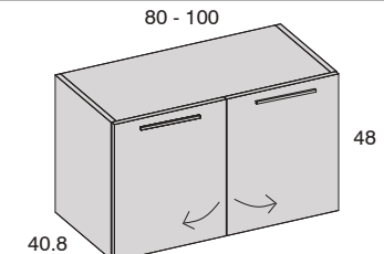
Módulo 2 puertas
