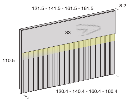
Cabezal regular Gap con plafón IZQUIERDA
