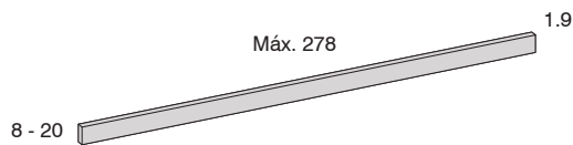
Tapeta 4 cantos chapados
