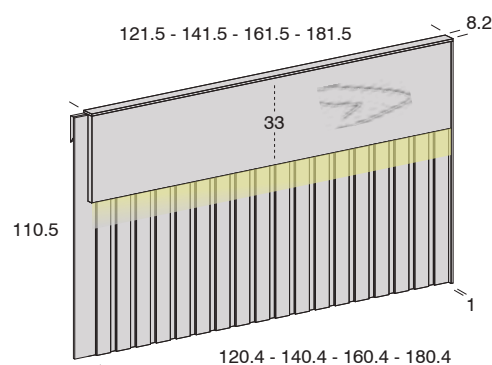
Cabezal regular Gap con plafón DERECHA
