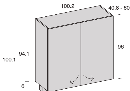
Altijo puente 2 puertas batientes
