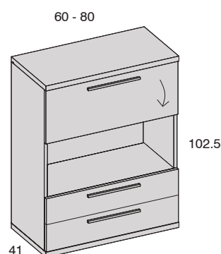
Chifonier 2 cajones + hueco + puerta abatible
