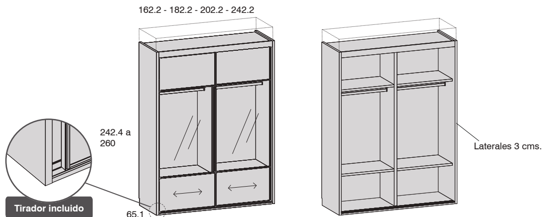
Armario 2 puertas correderas 3 plafones (plafón central cristal)
