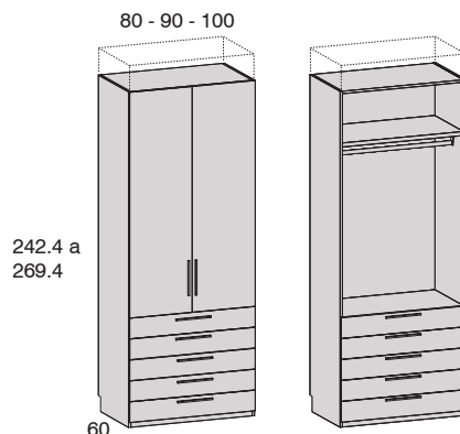
Armario 2 puertas + 5 cajones
