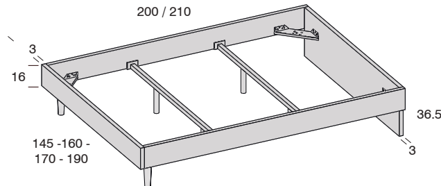
Aro Basic con patas de madera
