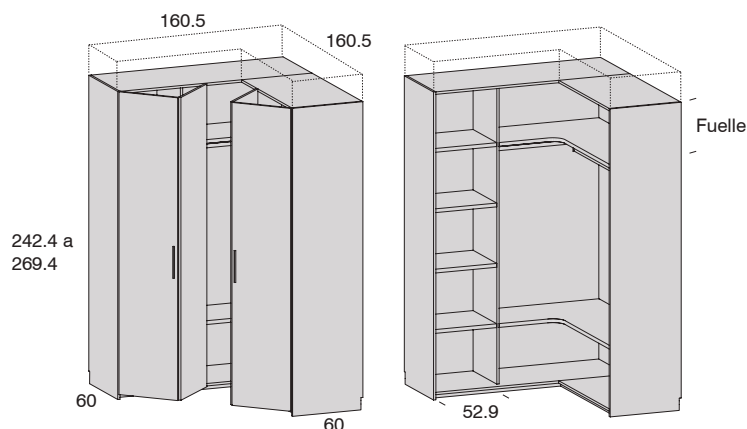
Armario rincón 4 puertas
