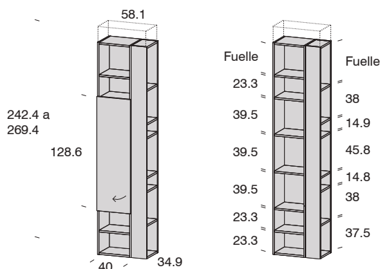
Terminal Troya armario IZQUIERDA
