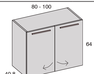
Módulo 2 puertas
