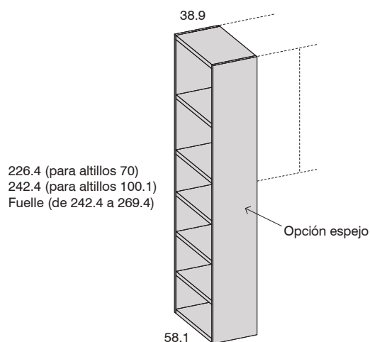
Montante estantería altillos
