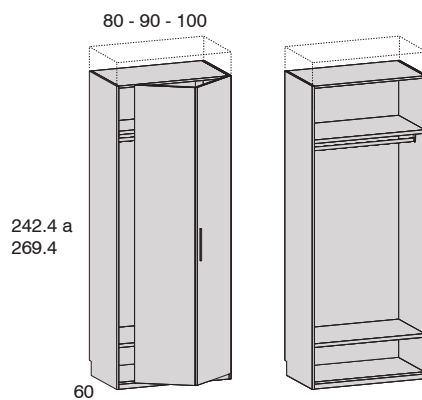
Armario 2 puertas DERECHA
