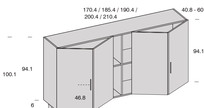
Altijo puente 4 puertas plegables
