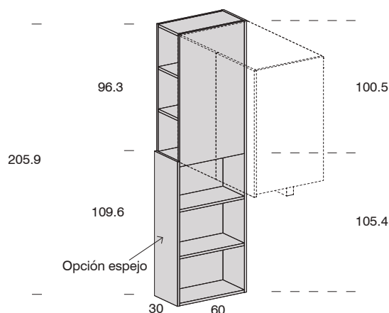
Montante para atillo 100.1 cms. alto IZQUIERDA
