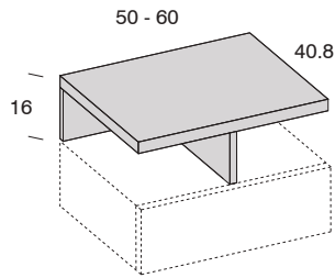
Base 2 huecos
