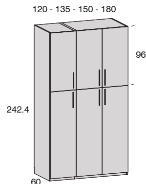
Armario 3 puertas + altillo 3 puertas IZQUIERDA
