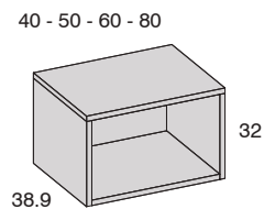
Mesita 1 hueco
