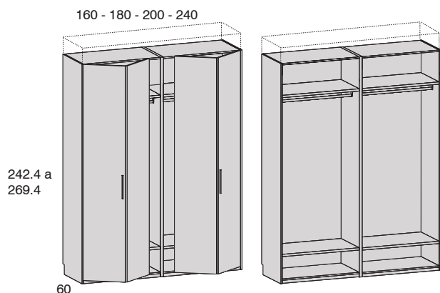
Armario 4 puertas
