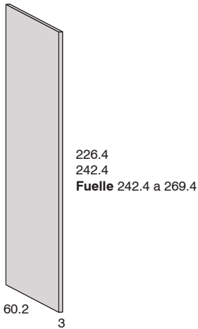
Sobrecostado armario 3 cms.
