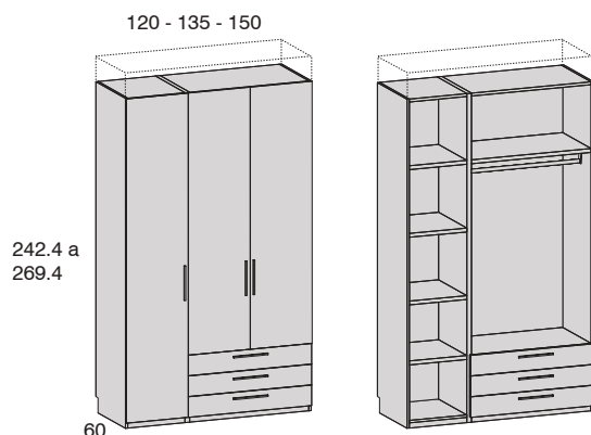
Armario 3 puertas IZQUIERDA + 3 cajones
