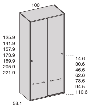
Armario Complet 2 puertas correderas ancho 100
