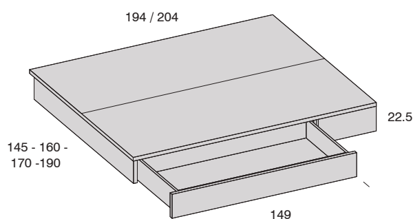
Base Etapa 1 cajón con ruedas
