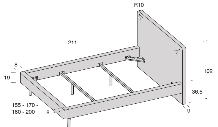
Cama tapizada Nett
