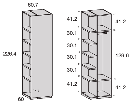
Armario terminal Open estantes IZQUIERDA
