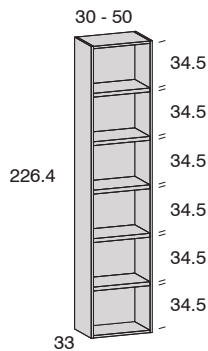
Librería terminal con trasera
