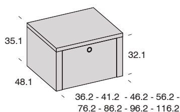
Cajonera interior 1 cajón doble
