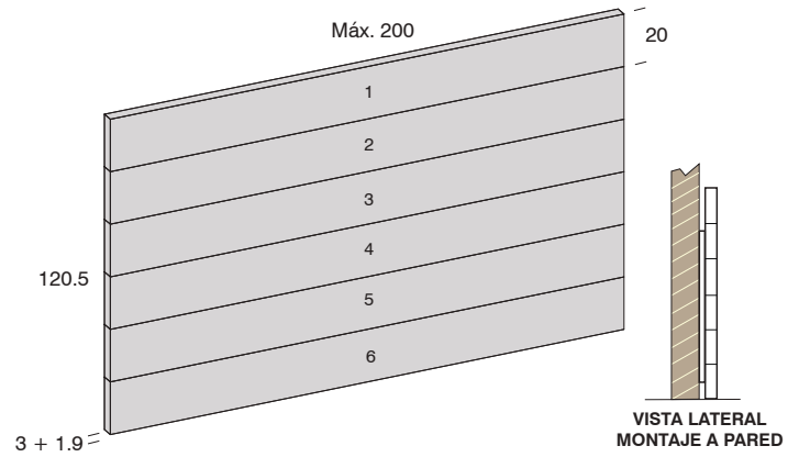
Cabezal Olimpia Horizontal de 120.5 cms.
