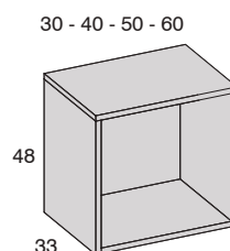
Galería Dorso fondo 33
