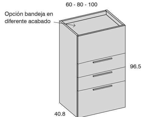
Chifonier Bandeja 1 cajón doble + 2 cajones + 1 cajón doble
