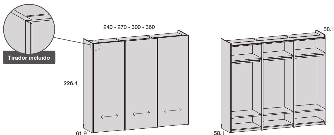
Armario 3 puertas correderas
