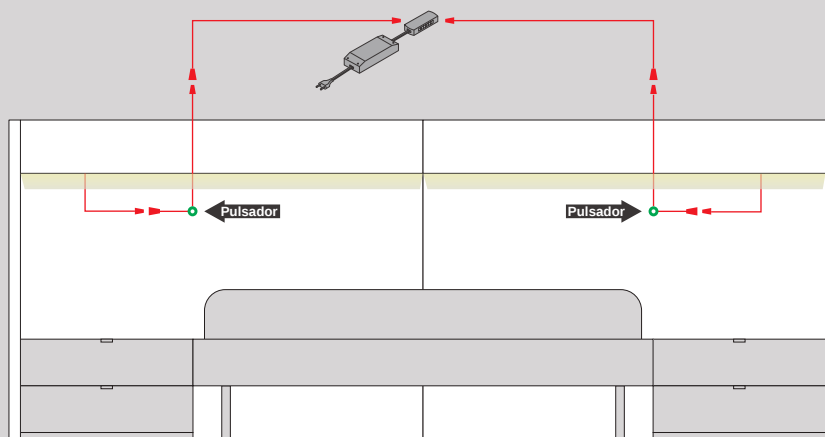
Esquema instalación leds en cabezal Horizon
