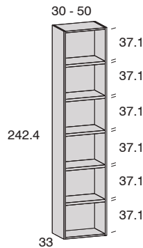
Librería terminal con trasera
