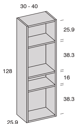
Galería Right fondo 25.9
