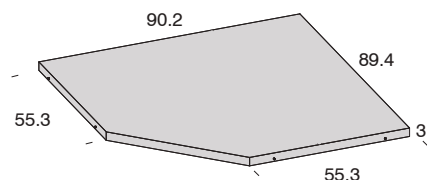
Estante interior para armario rincón DERECHA
