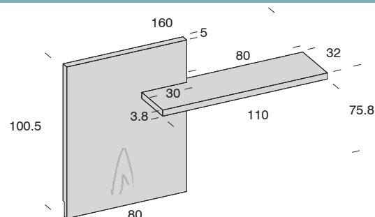
Panel + estante DERECHA
