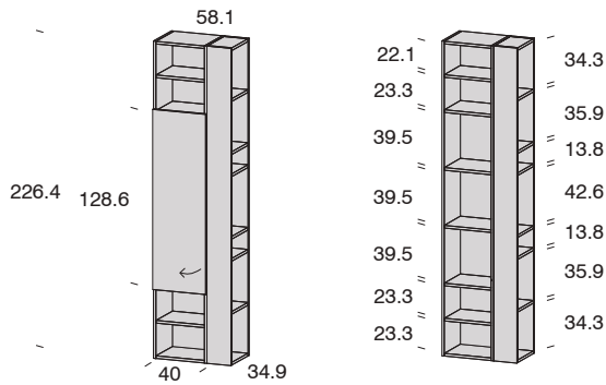
Terminal Troya armario IZQUIERDA
