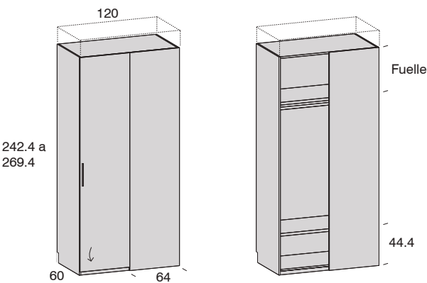
Armario ciego 1 puerta IZQUIERDA
