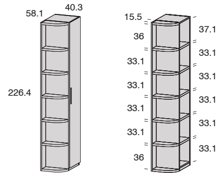
Armario terminal zapatero DERECHA
