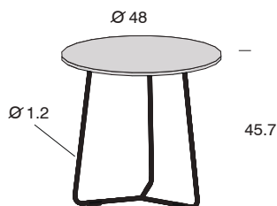
Mesita Redonda Subtile
