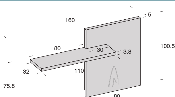
Panel + estante IZQUIERDA
