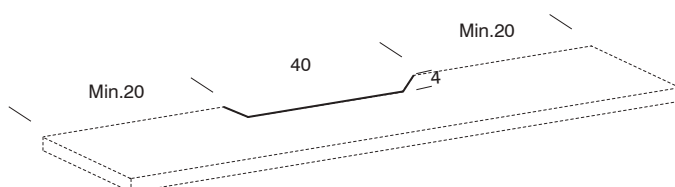
Rebaje trasero en sobre para pasar cables
