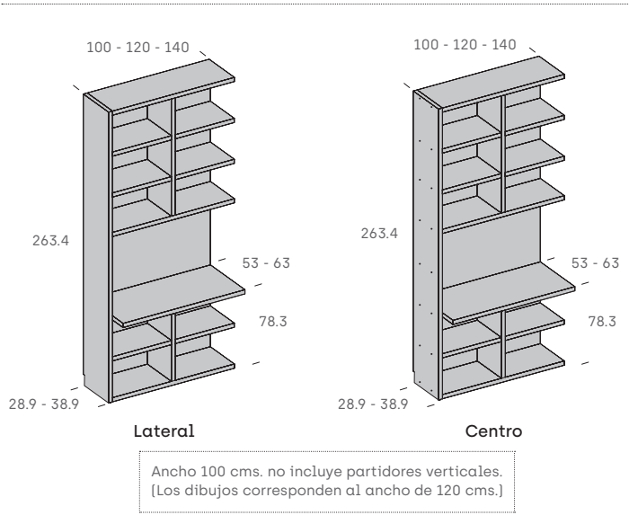
Detalle escritorio fijo cantos curvos
